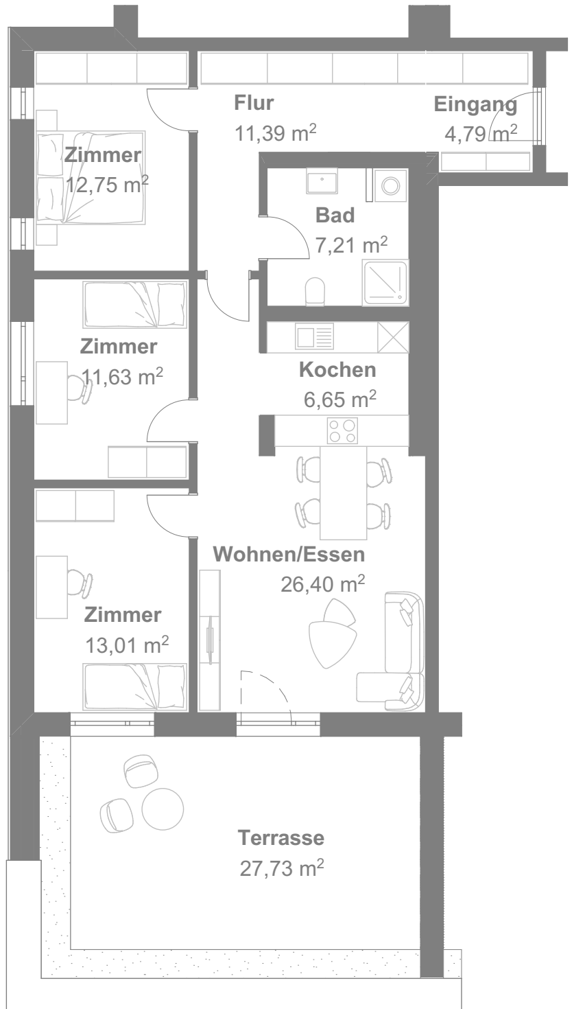
2. OBERGESCHOSS Typ III
